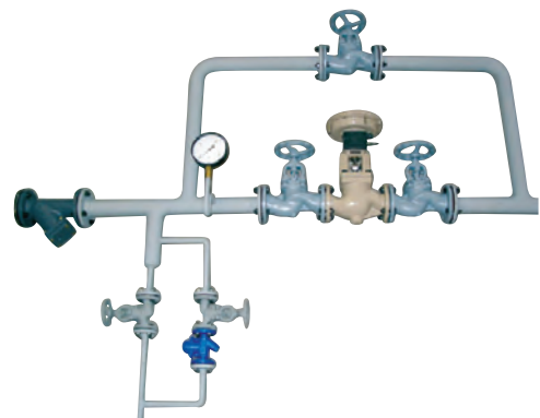
Dampfdosiereinheit mit elektro-pneumatischem Ventil DD - fertig verrohrt
