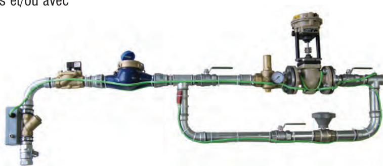
Unité de dosage d'eau avec valve électro-pneumatique DE- assemblage fini
